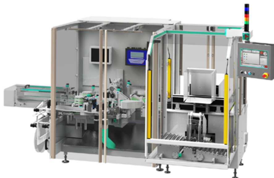
Track-Pack , состоящий из этикетировочной машины BL-A415 и укладчика в короба PS 300
