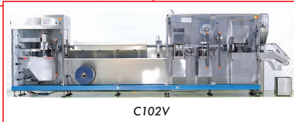
Блистерная машина PG EXCEL
